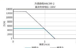
■ 力-速度曲线
