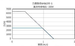
■ 力-速度曲线
